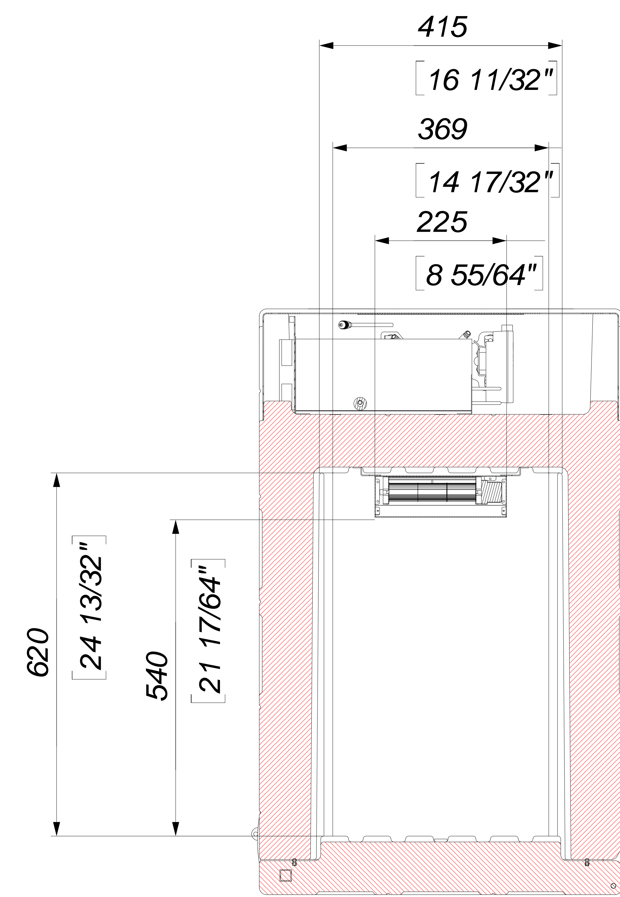
Sezione F-F SCALE 1 : 4
