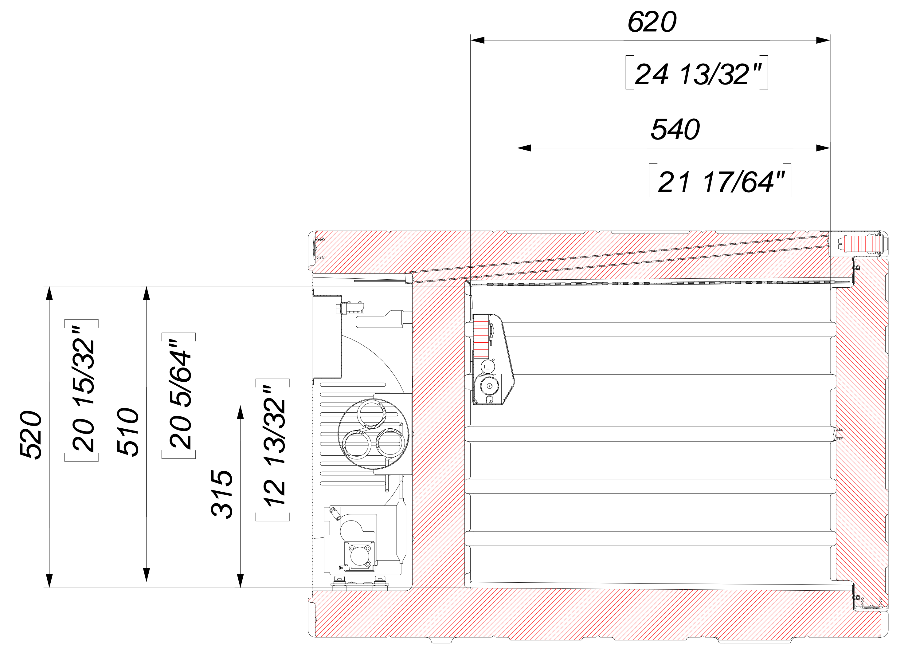
Sezione E-E SCALE 1 : 4
